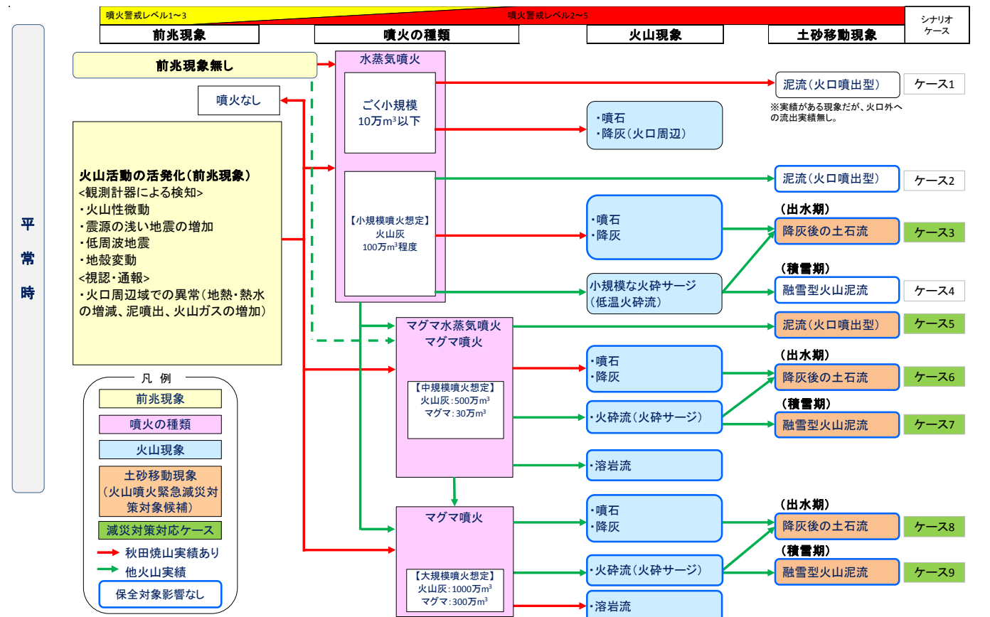
図-2 秋田焼山イベントツリー
